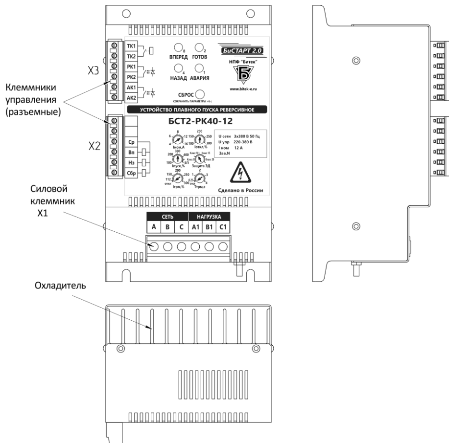
Рисунок 1 - Внешний вид пускателя БСТ2-РК40-12
