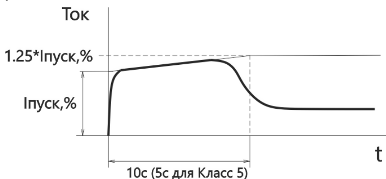
Рисунок 8 Плавный пуск с ограничением тока
