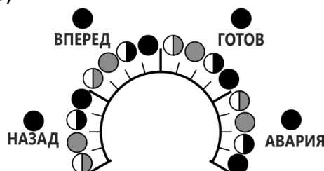
Рисунок 6 Индикация положения потенциометра
