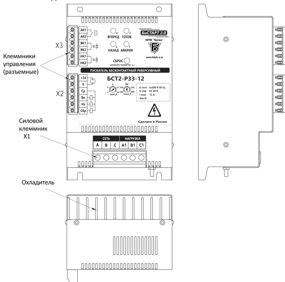
Рисунок 1 - Внешний вид пускателя БСТ2-Р33-12
