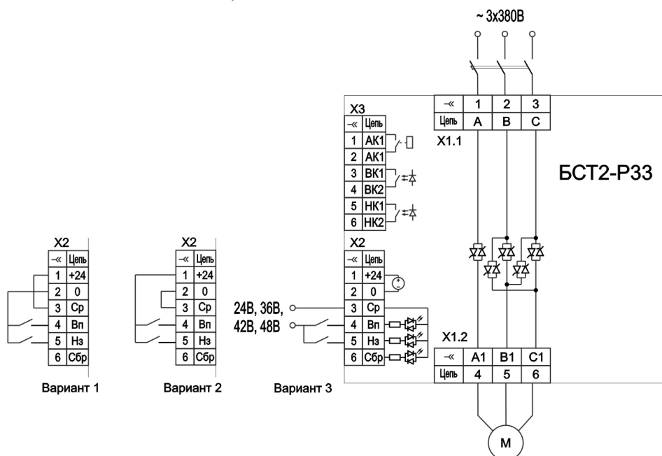
б) БСТ2-Р33
