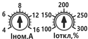
Рисунок 4 Органы настройки БСТ2
