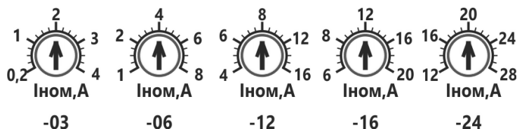
Рисунок 5 Диапазоны настройки Ином для моделей 03А, 06А, 12А, 16А, 24А
