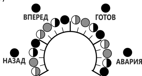
Рисунок 6 Индикация положения потенциометра
