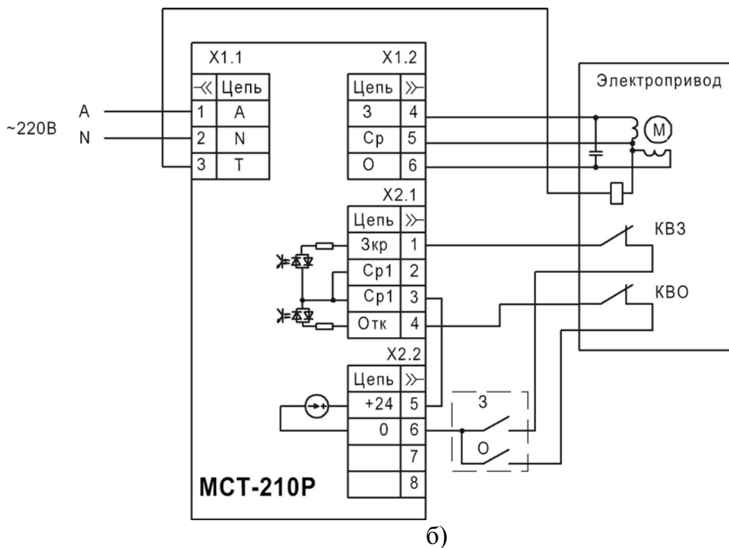
Рисунок 2 –Пример схемы подключения а) МСТ-110P б) МСТ-210P
