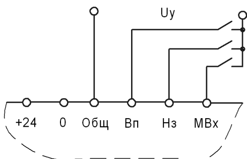
Рисунок 2 – Примеры схем подключения пускателя
