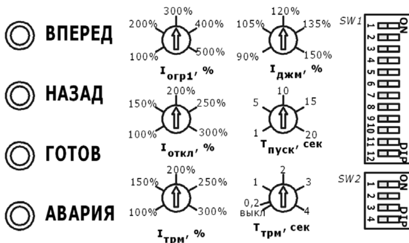
б) БСТ-ххР/380-х1
